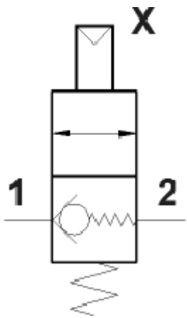
2/2 blokkeerventiel symbool
